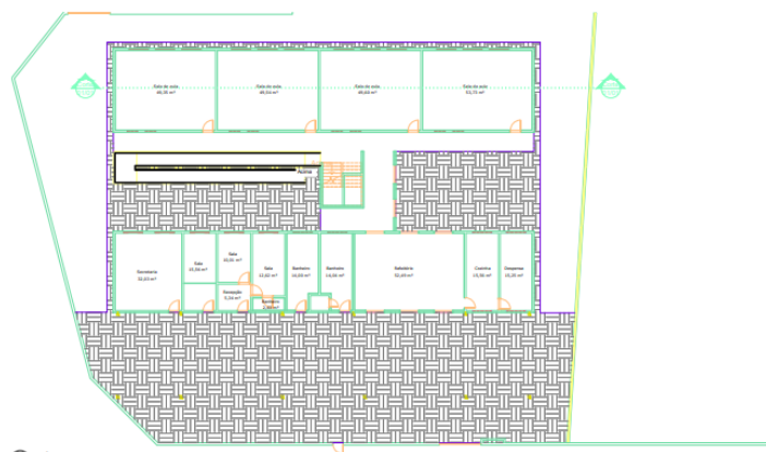
1. TÉRREO ESCALA: 1:100
